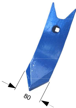
„Mulch-Mix 80“ Scharspitze
